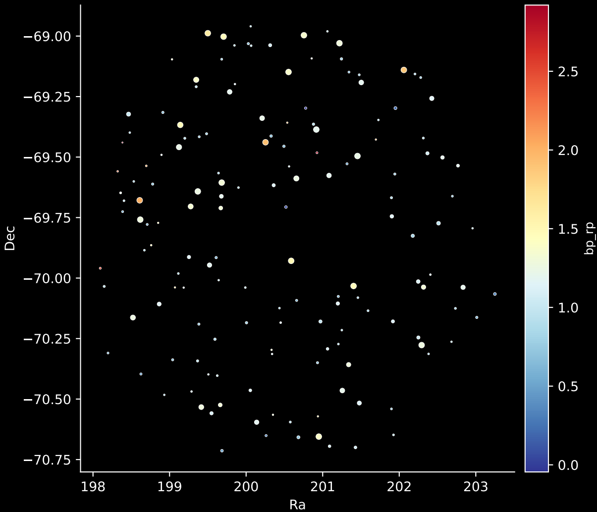
APOGEE DR17 Field: [280-26-O_TESS] Stars: 156
