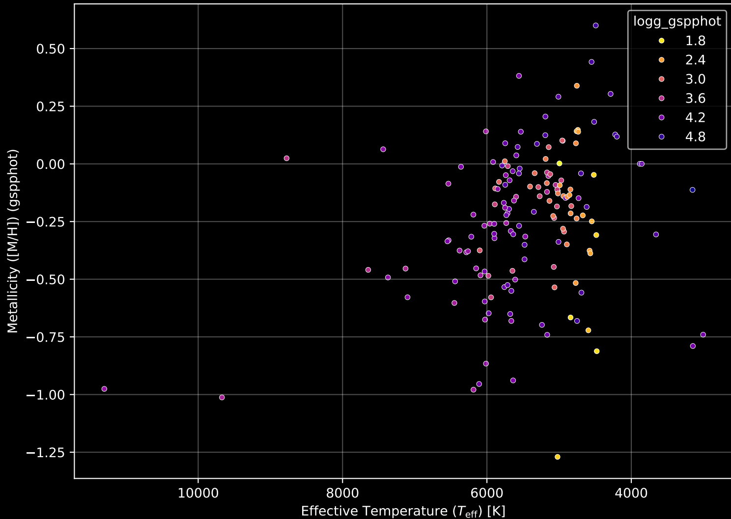
APOGEE DR17 Field: [280-26-O_TESS] Stellar Population Parameters (n= 156)
