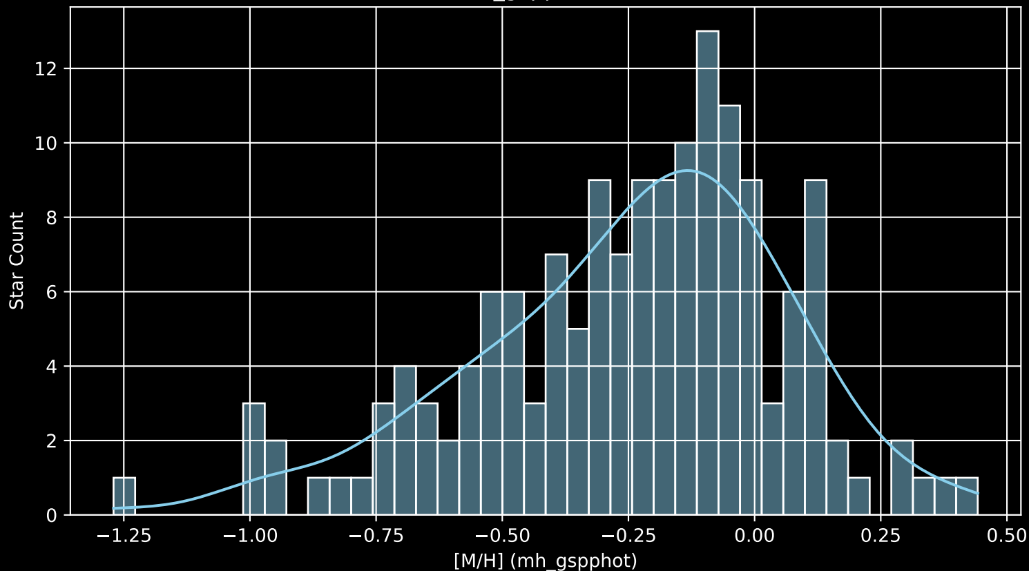
APOGEE DR17 Field: [280-26-O_TESS [M/H] (mh_gspphot) (n= 155)
